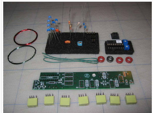
Antennentuner
