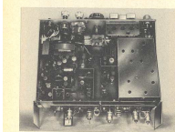
Bild 90. Innenansicht der 2-m-Station von DL9IW
