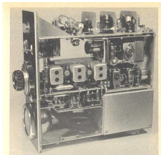
Bild 64. Innenansicht der 2-m-Station von DL9AL mit Zf-Baustein
