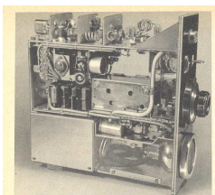
Bild 67. 2-m-Station von DL9AL, Innenansicht von der Tuner-Seite
