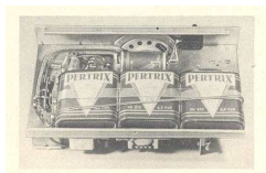
Bild 81. Unterbringung der Batterien unter dem Chassis
