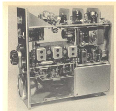
Bild 88. Innenansicht der 2-m-Station von DL9AL mit Zf-Baustein
