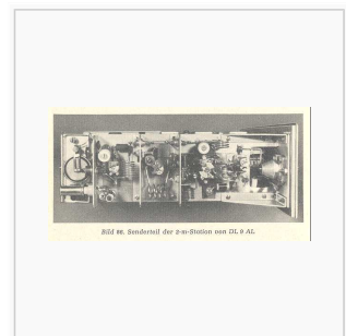
Senderteil DL9AL
