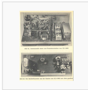
Innenansicht der DJ5MM 2m Transistorstation
