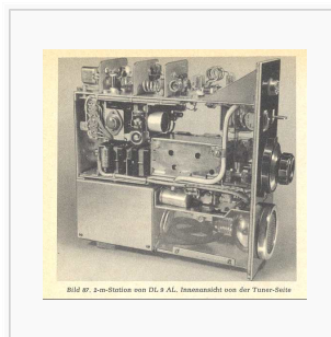
2m Station von DL9AL , Tunerteil
