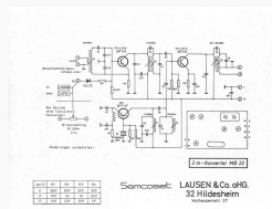
MB-22 Konverter Schaltbild
