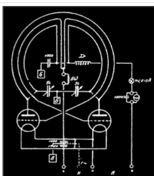
Gegentaktsender
