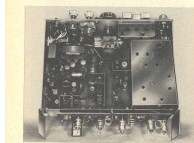
Bild 88. Innenansicht der 2-m-Station von DL9AL
