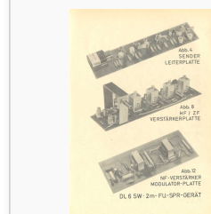
Leiterplatten Abb.
