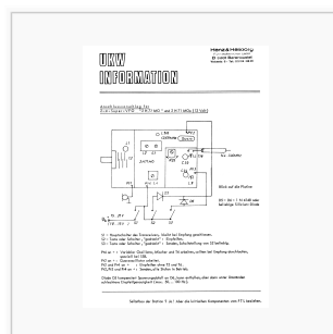
Anschlussvorschlag VFO
