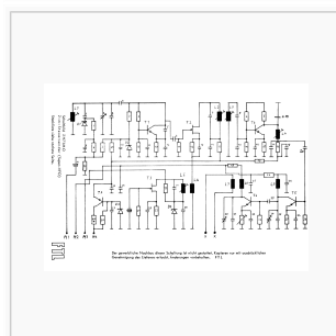
Schaltbild
