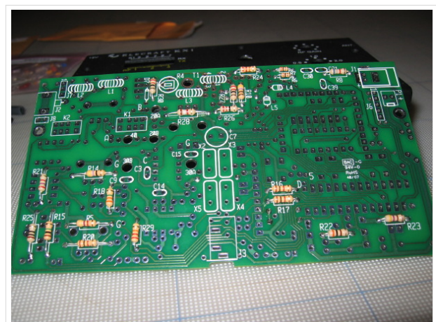
Hauptplatine
