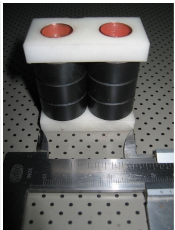
Aufbau Transformator
