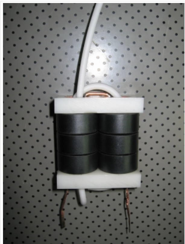
Aufbau Transformator
