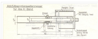
X Band Wellenmesser von OE1RVW nach Unterlagen der RSGB
