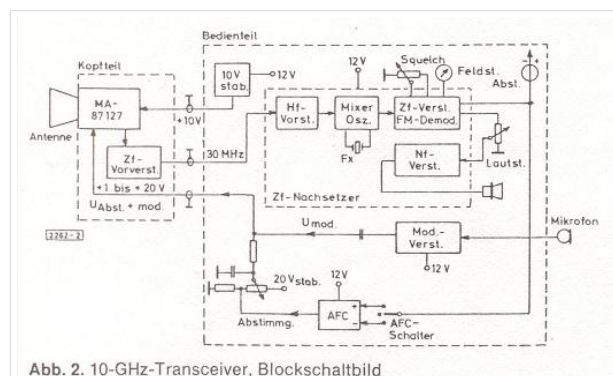
Blockschaltbild 3cm WBFM Transceiver mit MA87127
