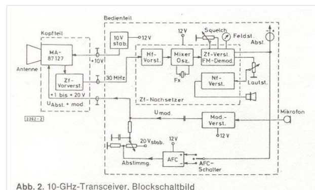
Blockschaltbild 3cm WBFM Transceiver mit MA87127
