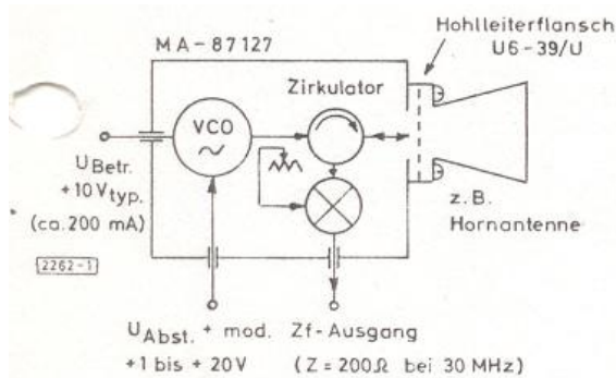
Abb. 1. Gunnplexer; Blockschaltbild
