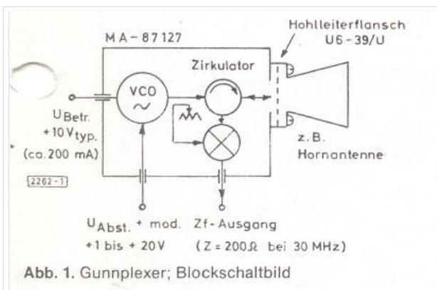
Blockschaltbild MA87127
