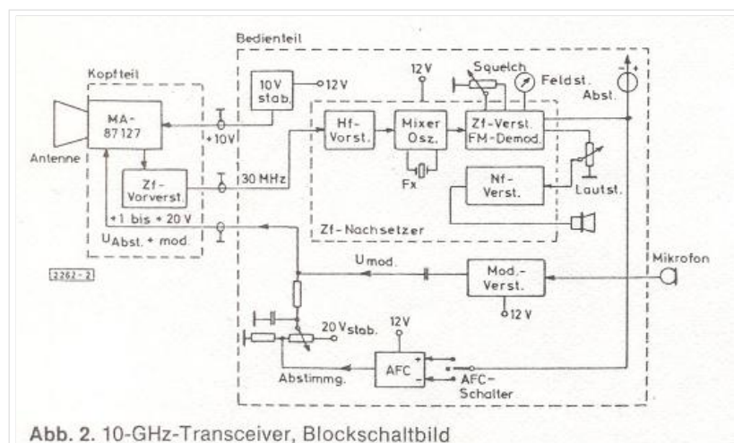
Blockschaltbild 3cm WBFM Transceiver mit MA87127
