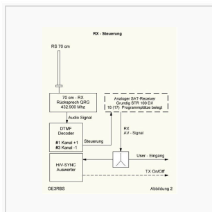
RX Steuerung
