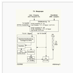
TX Baugruppe
