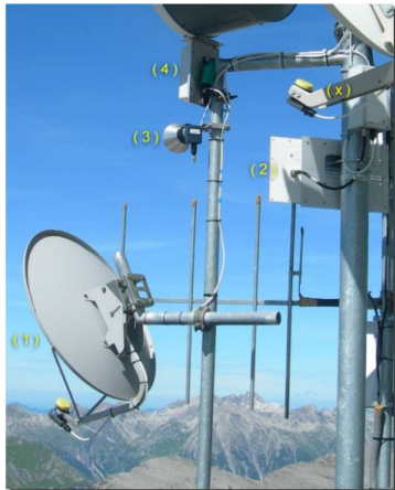
OE7XLT Empfangsantennen
