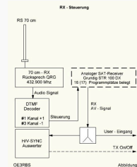
RX Steuerung
