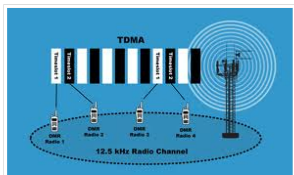
Zeitschlitzverfahren
