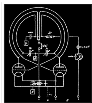
Gegentaktssender
