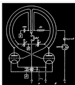
Gegentaktssender
