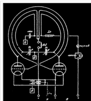
Gegentaktsender
