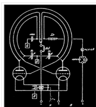
Gegentaktssender
