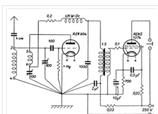
Audionsschaltung
