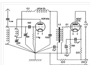
Audionschaltung
