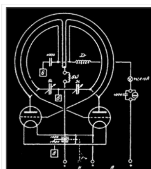
Gegentaktsender
