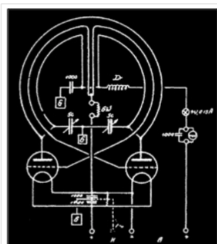
Gegentaktssender
