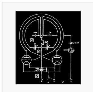
Gegentaktsender
