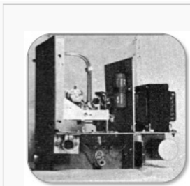
Wallmann Konverter Seitenansicht
