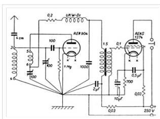
Audionsschaltung
