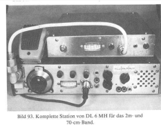
Bild 93. Komplett Station von DL6MH für das 2m- und 70-cm-Band.
