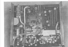
Bild 92. Innenansicht des 70-cm-Zusatzgerätes von DL 6 MH.
