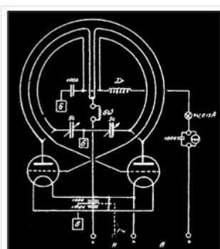
Gegentaktsender
