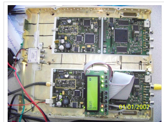
70cm ATV-Sender - Feldversuch im April 2010
