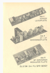
Zusammenbau Leiterplatten
