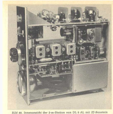
2m Station von DL9AL mit Zf-Baustein
