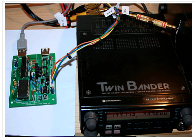
Die Platine wurde in ein Europakartengehäuse aus Aluminium eingebaut. Ein Metallgehäuse ist wichtig, da der uP ziemlich stark auf seiner Quarzfrequenz und Vielfachen strahlt.
