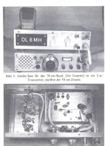
Bild 94. Innensicht des in Bild 3 gezeigten Transceiver-Ordnens. Links der Frequenzwandler, rechts der Transmitter nach DL 6 MH.
