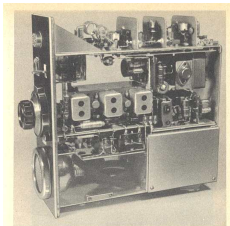
Bild 88. Innenansicht der 2-m-Station von DL 9 AL mit Zf-Baustein
