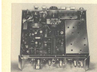
Bild 90. Innenansicht der 2-m-Station von DL 9 AL
