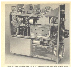
Bild 89. 2-m-Station von DL 9 AL, Innenansicht von der Tuner-Seite
