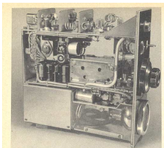
Bild 87. 2-m-Station von DL9AL. Innenseite von der Tuner-Seite
