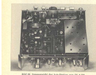
Bild 88. Innenseite der 2-m-Station von DL9AL
