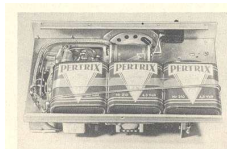
Bild 41. Unterbringung der Batterien unter dem Chassis
