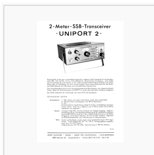
Tragbares UKW Funkgerät für SSB/AM /CW (1966)
