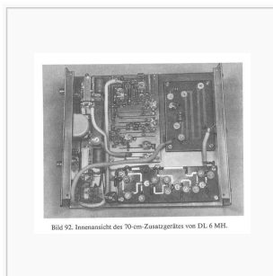
Transverter für 70cm nach DL6MH
