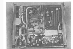
Bild 92. Innenansicht des 70cm-Zusatzgerätee von DL 6 MH.
