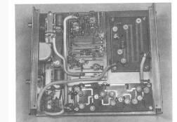
Bild 92. Innenansicht des 70-cm-Zusatzerfies von DL 6 MH.
