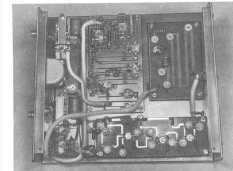
Bild 92. Innenansicht des 70cm-Zusatzerweiterung von DL 6 MH.
