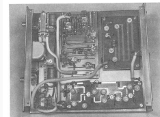
Bild 92. Innenansicht des 70cm-Zusatzerätes von DL 6 MH.
