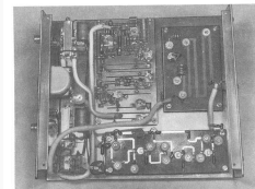
Bild 92. Innenansicht des 70cm-Zusatzerätes von DL 6 MH.
