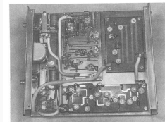
Bild 92. Innenansicht des 70cm-Zusatzerweiterungsgliedes von DL 6 MH.
