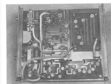
Bild 92. Innenseite des 70cm-Zusatzerfües von DL 6 MH.
