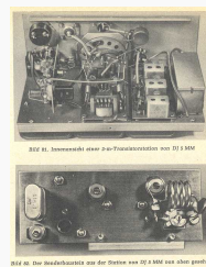
Innenansicht der 2m Transistorstation
