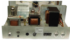
Minix MTR 25 S Frontansicht
