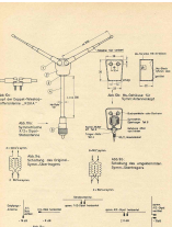
Abb. 5. Radiorezeptions-Apparat für den Funkdienst.
