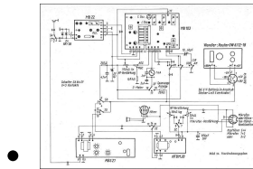
MB-103 Verdrahtungsplan
