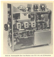
Bild 88. Innenansicht der 2-m-Station von DL9AL mit Zf-Baustein
